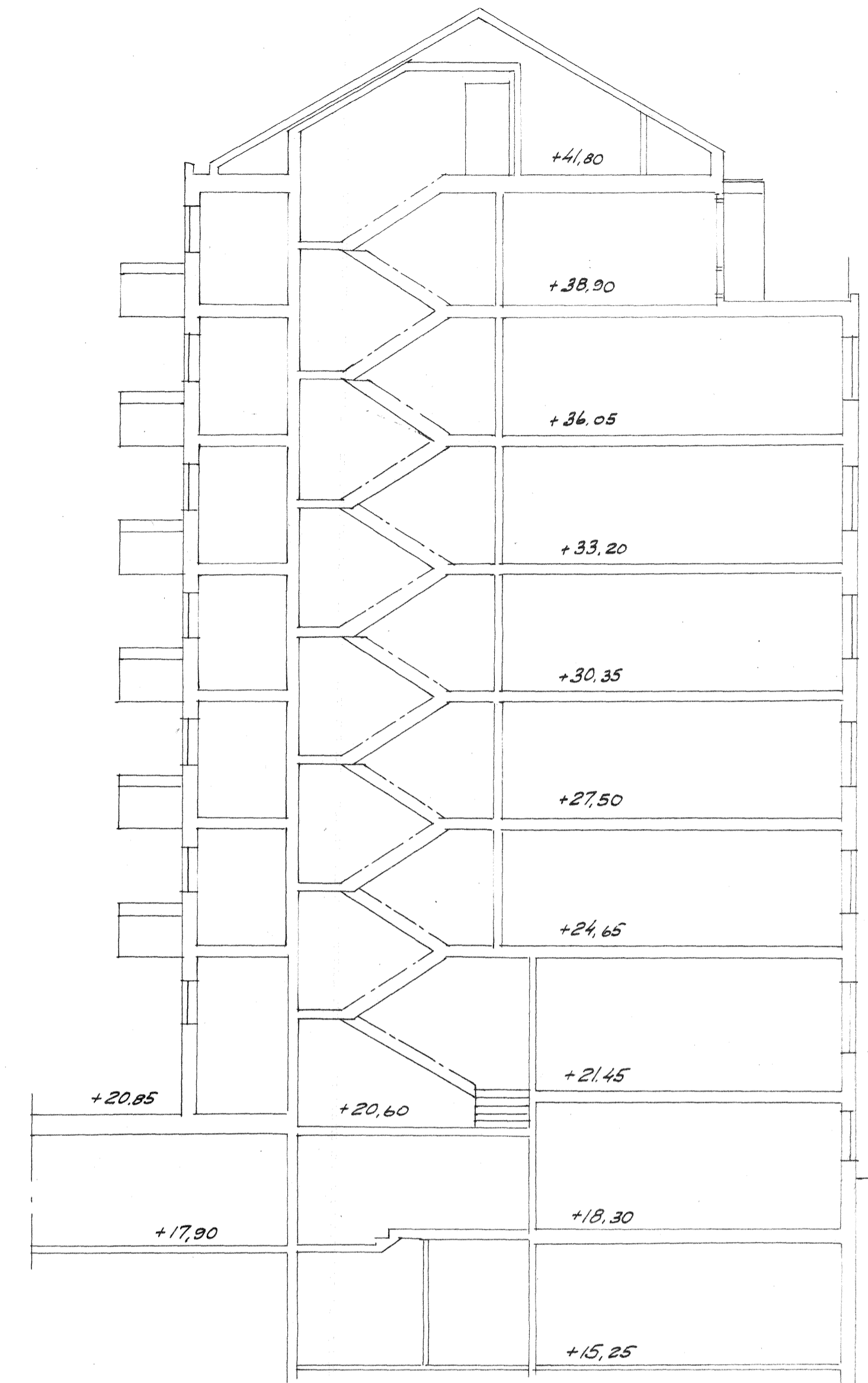
Sektion skala 1:100 dm 0 1 2 3 4 5 6 7 8 9 10 m
